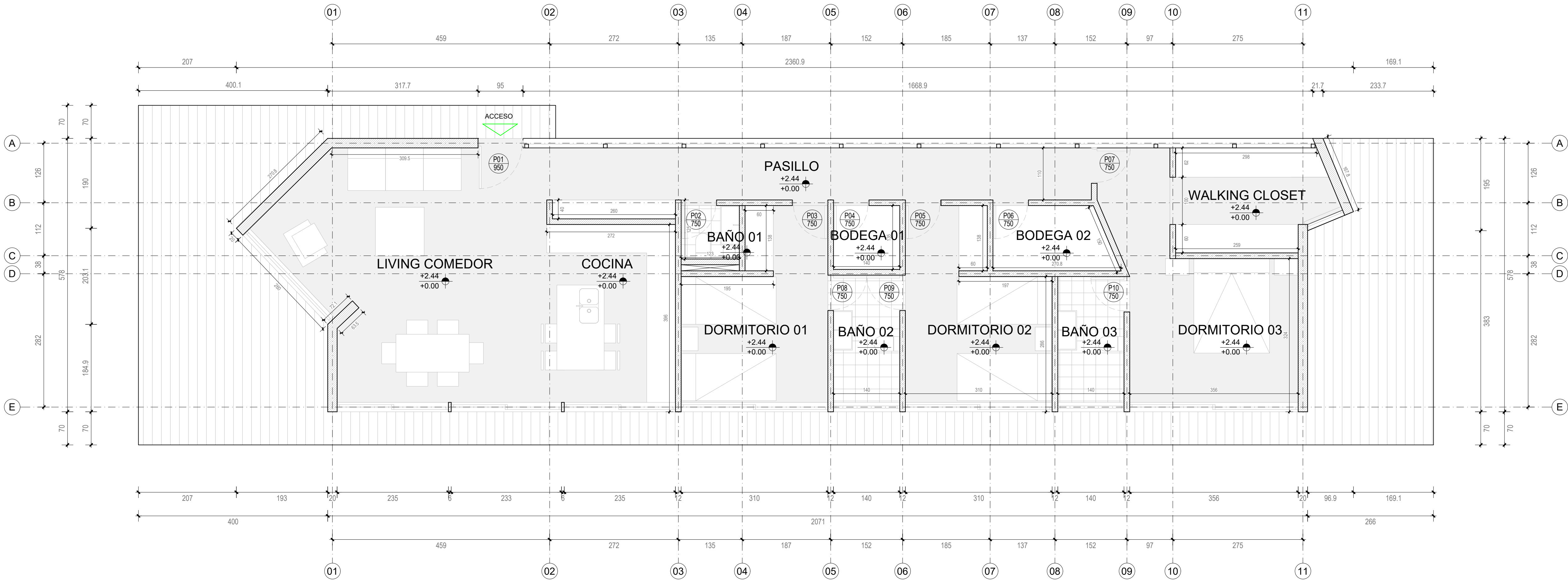
PLANTA DE ARQUITECTURA CASA C ESCALA 1:50
