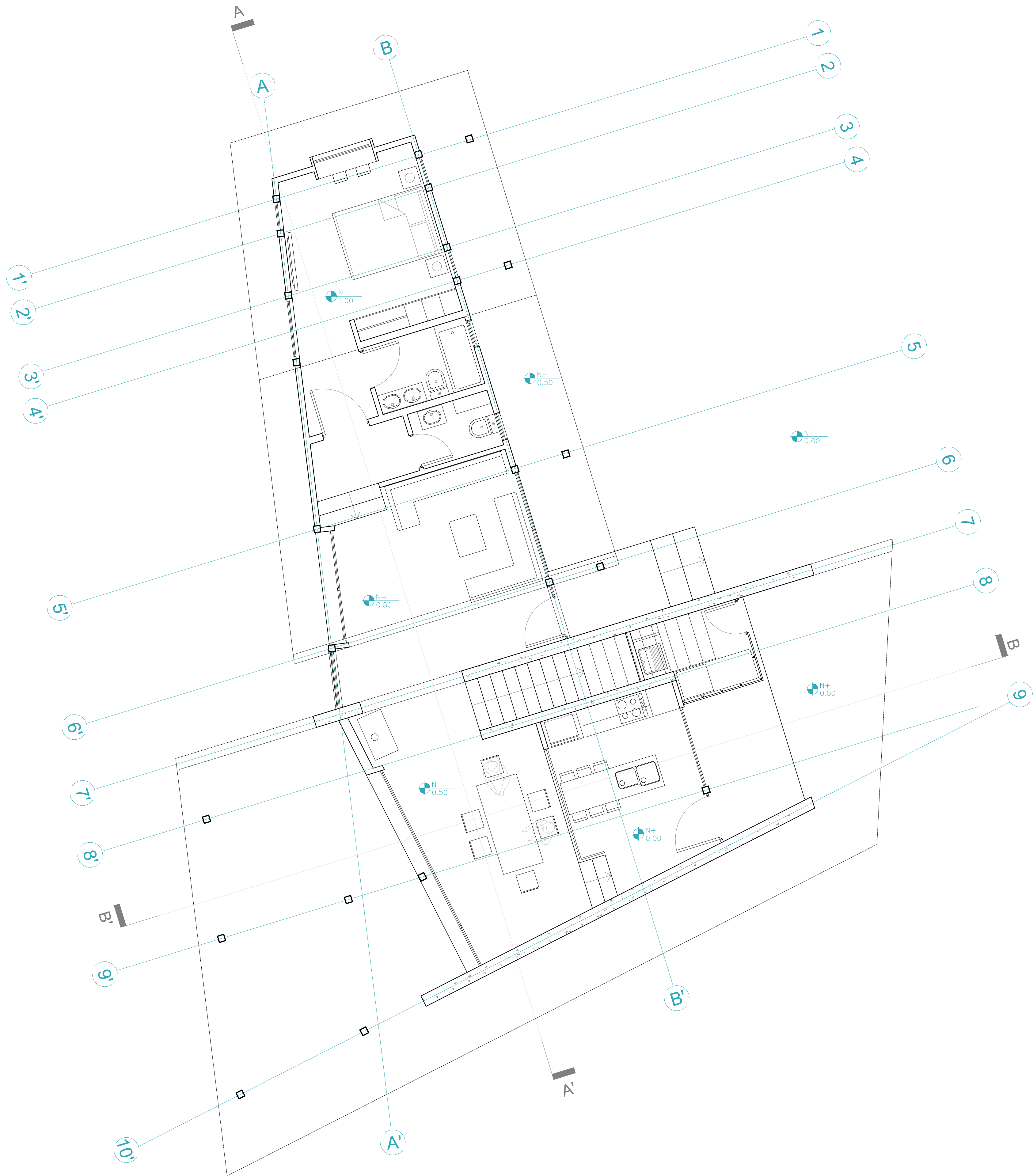
PLANTA PRIMER PISO ESCALA 1/50
