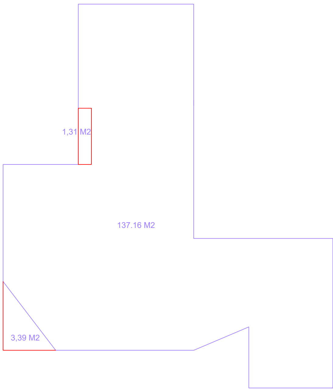
ESQUEMA DE SUPERFICIES PRIMER NIVEL SITUACIÓN PROPUESTA
