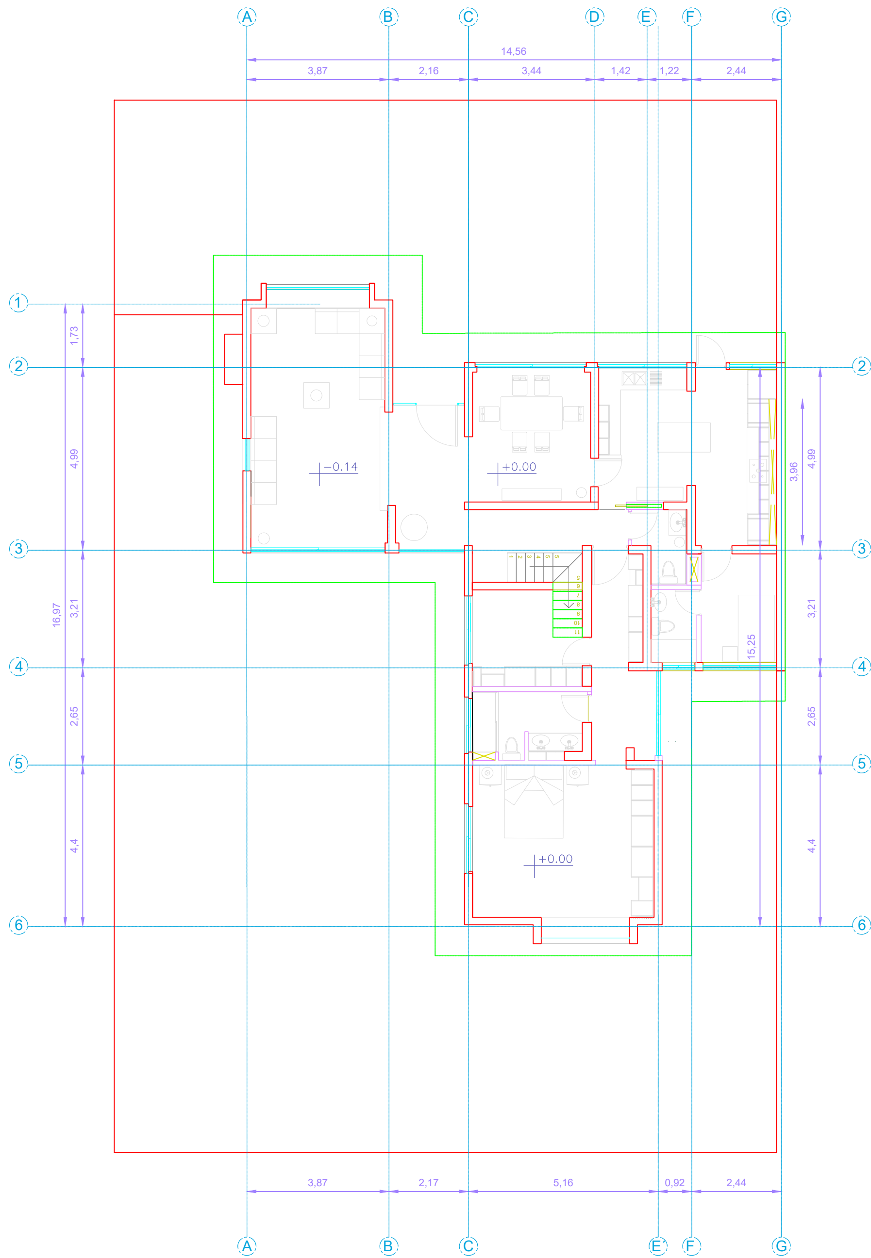
PLANTA PRIMER NIVEL EXISTENTE
